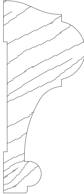
SCM 5046 1-1/2 X 3-1/2
