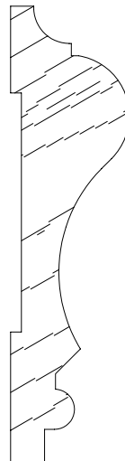
SCM 5049 11/16 X 2-5/8
