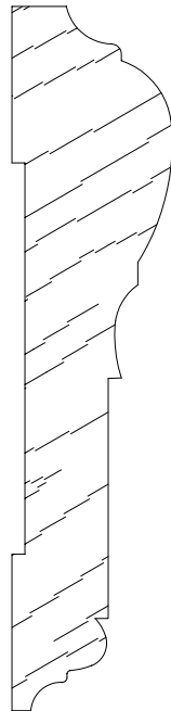
SCM 5024 3/4 X 3-3/8
