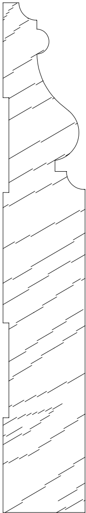
SCM 1056 7/8 X 5-3/8
