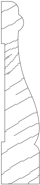
SCM 1021 11/16 X 3-1/4
