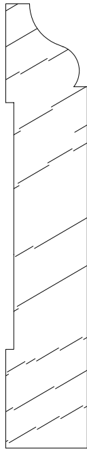
SCM 1057 5/8 X 3-3/8
