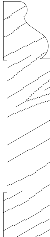
SCM 1034 13/16 X 4
