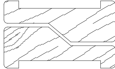
SCM 14007D 11/16 X 1-7/8
