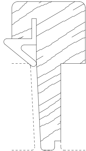
SCM 14004FW 1-1/2 X 3
