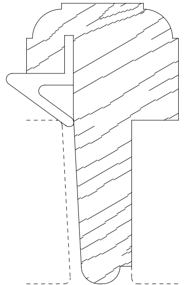
SCM 14002RW 1-5/8 X 3
