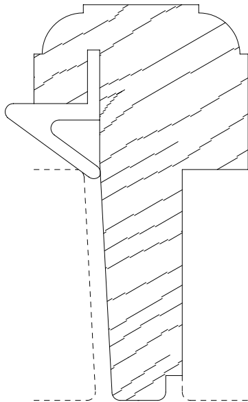
SCM 14002FW 1-5/8 X 3
